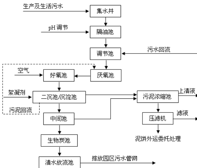
废水预处理工艺流程图
